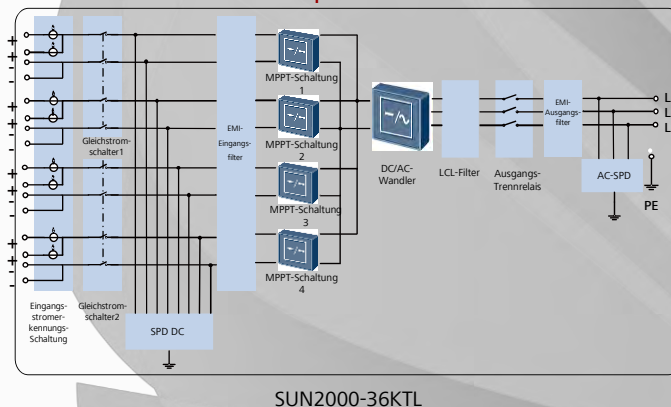
Schaltplan
